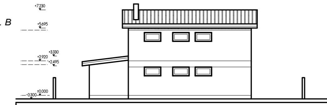
POHLAD ZADNÝ
